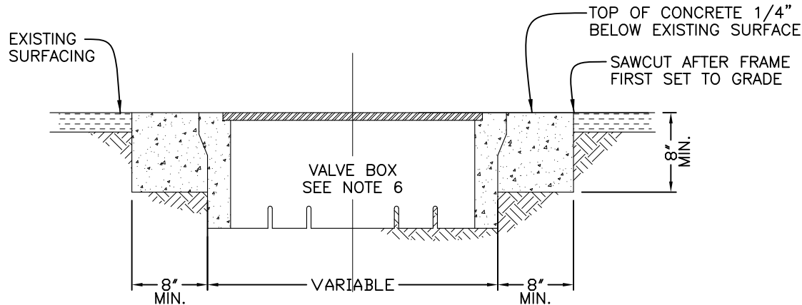
ELEVATION N.T.S.
